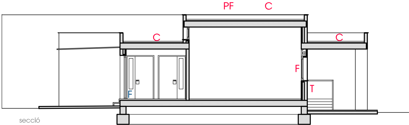
secció transversal
